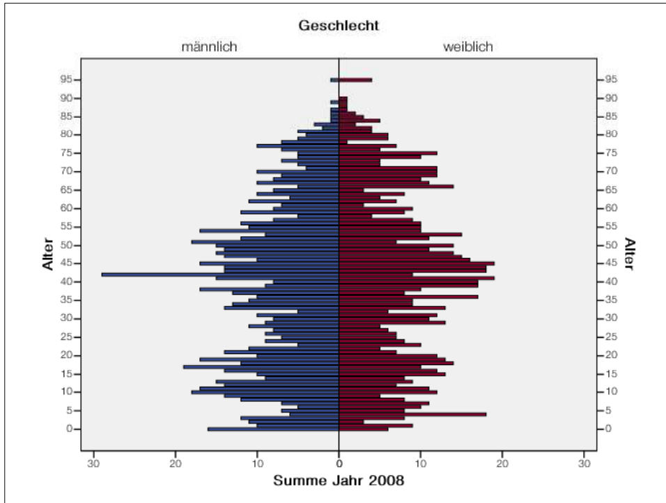
Abbildung 1: Bevölkerungsstand Unterreit 2008
