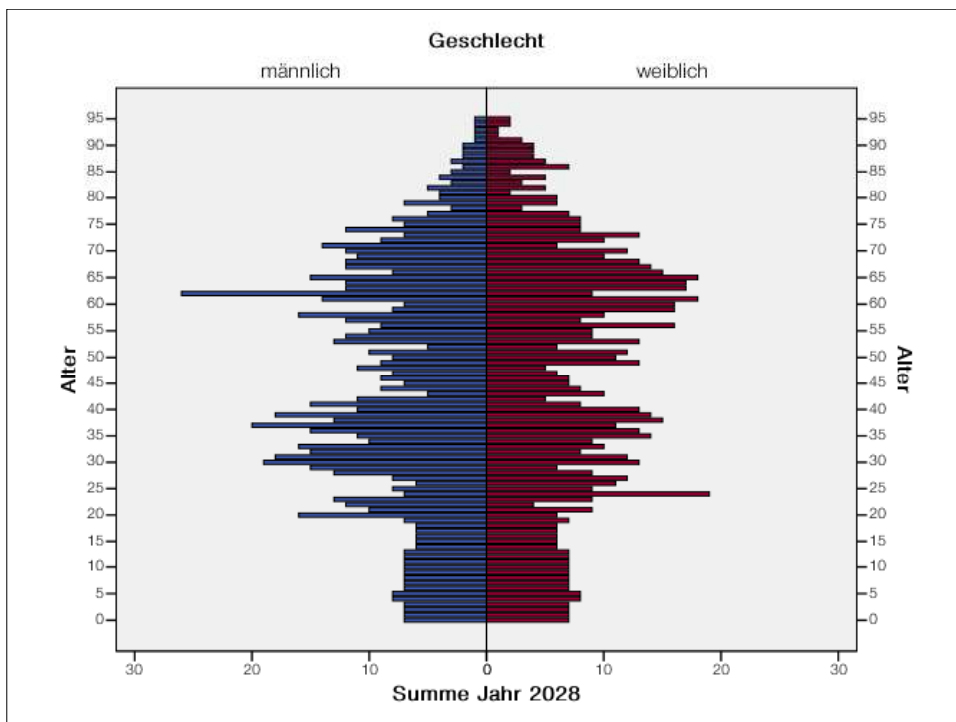
Abbildung 2: Prognose Unterreit 2028
