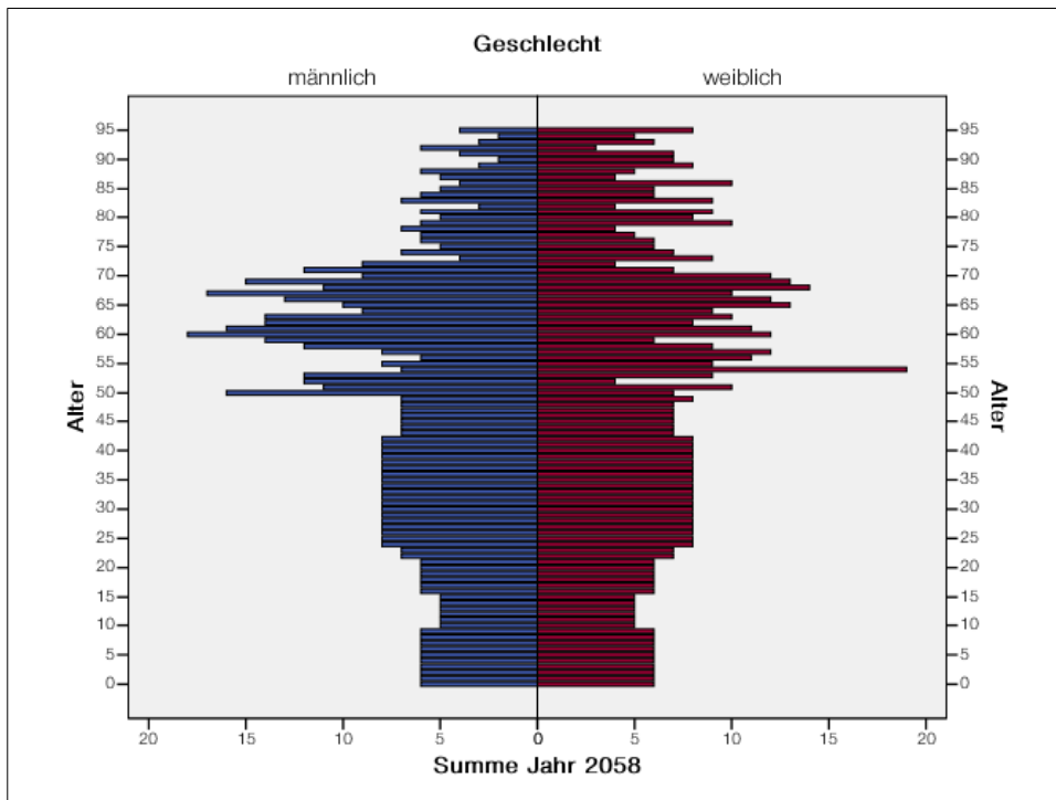
Abbildung 3: Vorausberechnung Unterreit 2058
