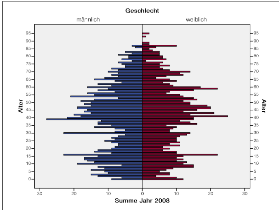
Abbildung 1: Bevölkerungsstand Maitenbeth 2008
