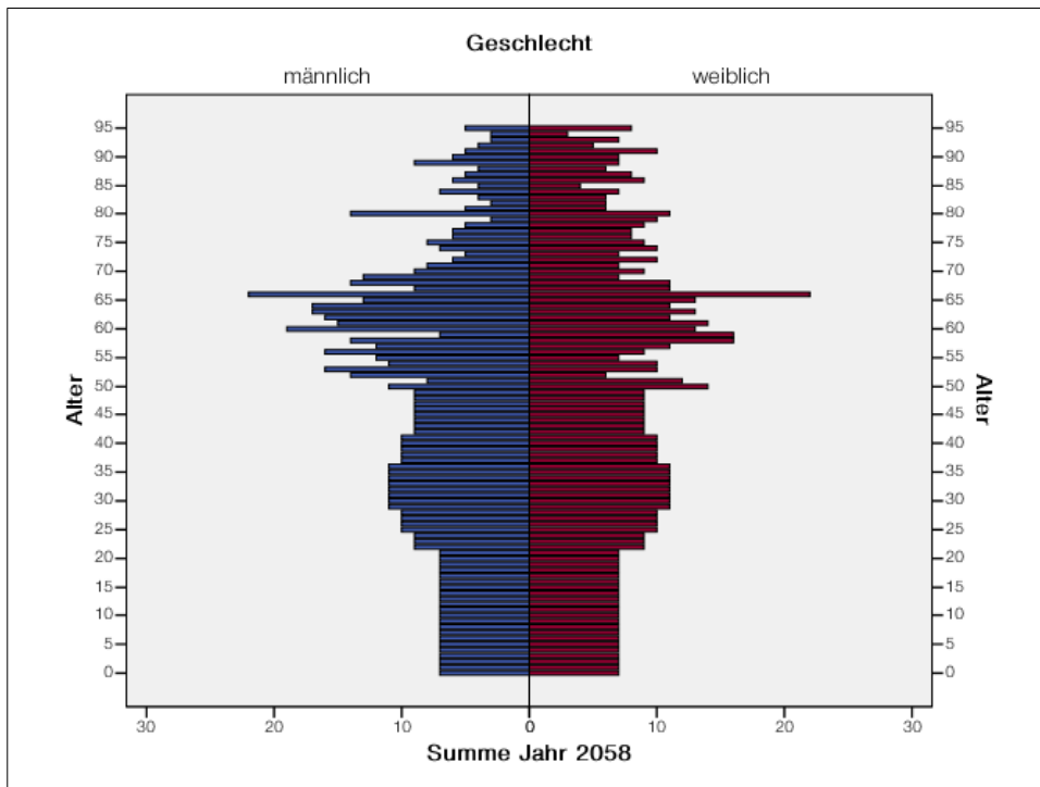
Abbildung 3: Vorausberechnung Maitenbeth 2058
