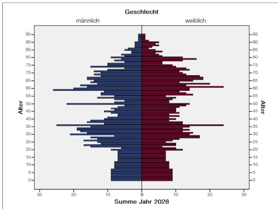
Abbildung 2: Prognose Maitenbeth 2028
