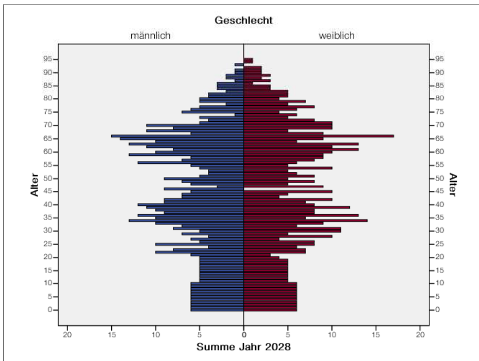
Abbildung 2: Prognose Eggkofen 2028
