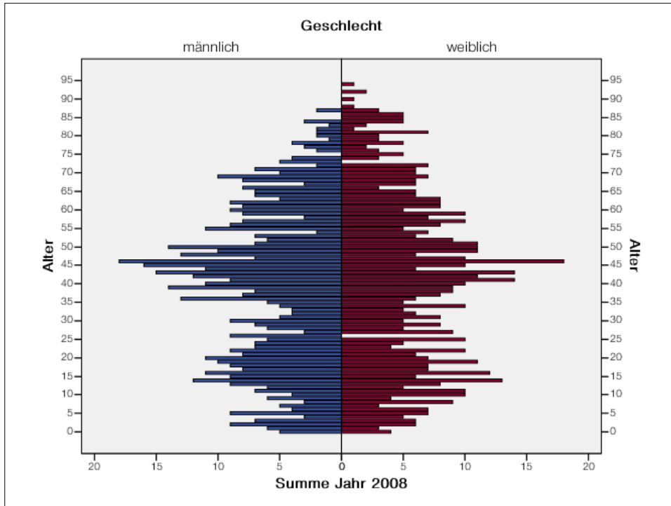
Abbildung 1: Bevölkerungsstand Eggkofen 2008
