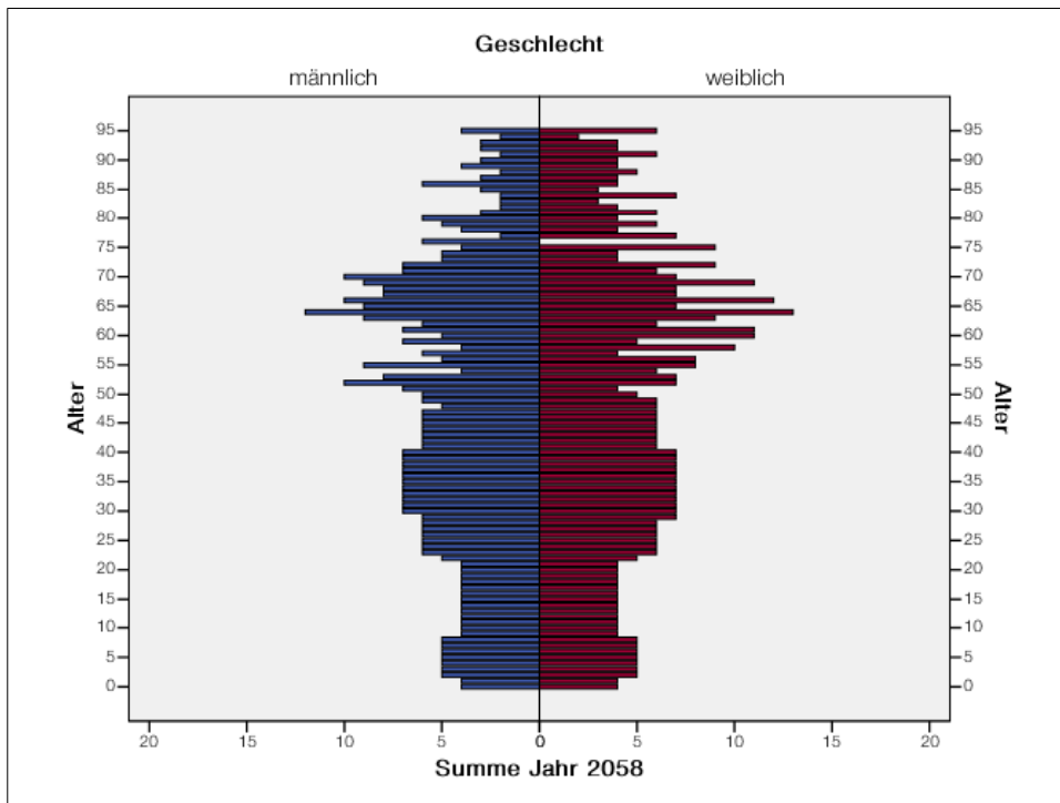
Abbildung 3: Vorausberechnung Eggkofen 2058
