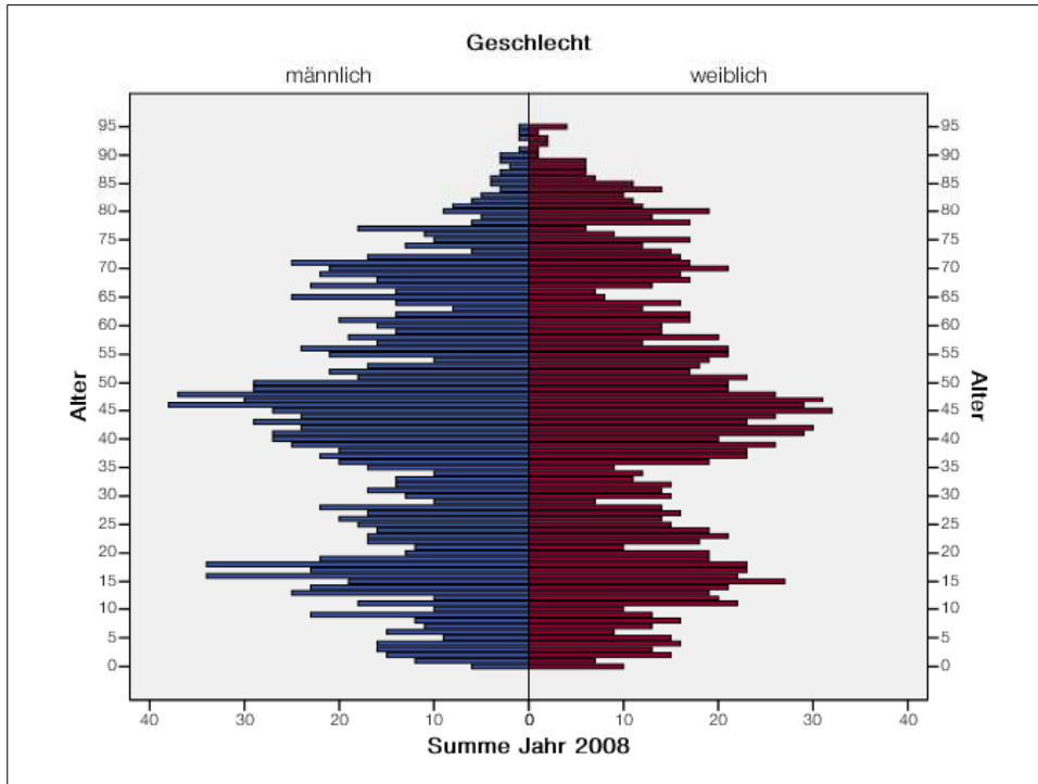
Abbildung 1: Bevölkerungsstand Buchbach 2008
