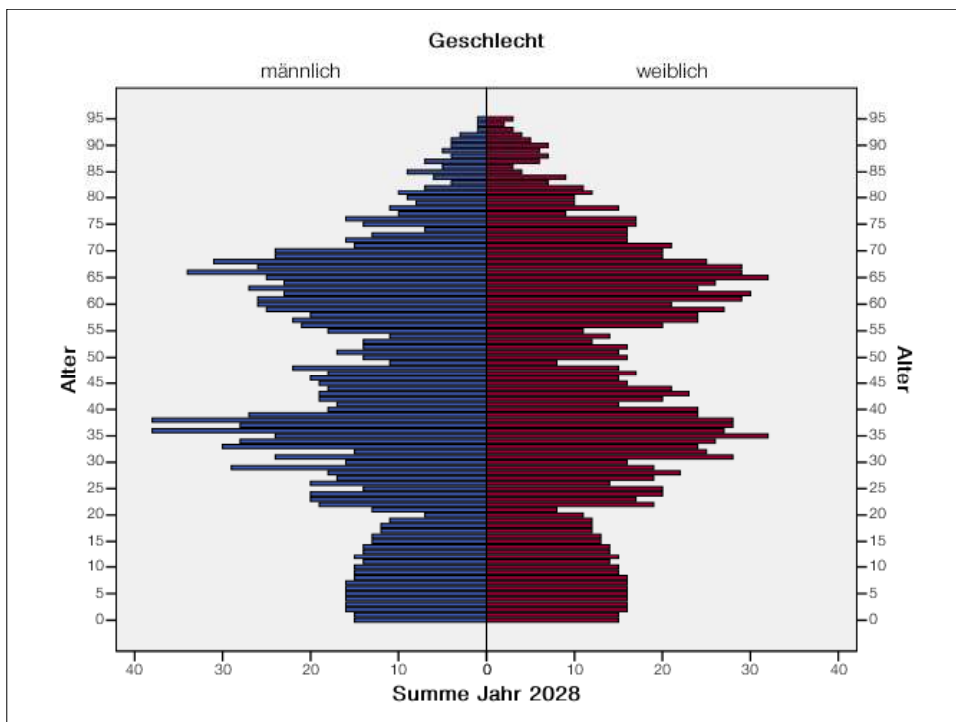
Abbildung 2: Prognose Buchbach 2028
