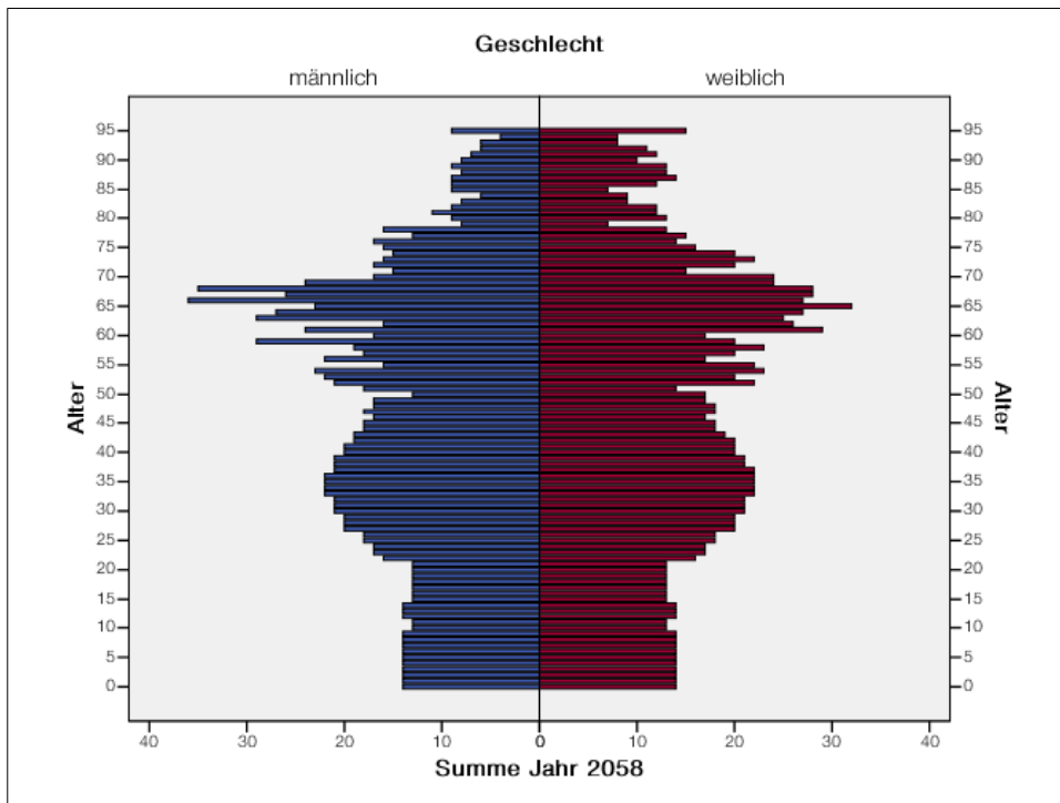
Abbildung 3: Vorausberechnung Buchbach 2058
