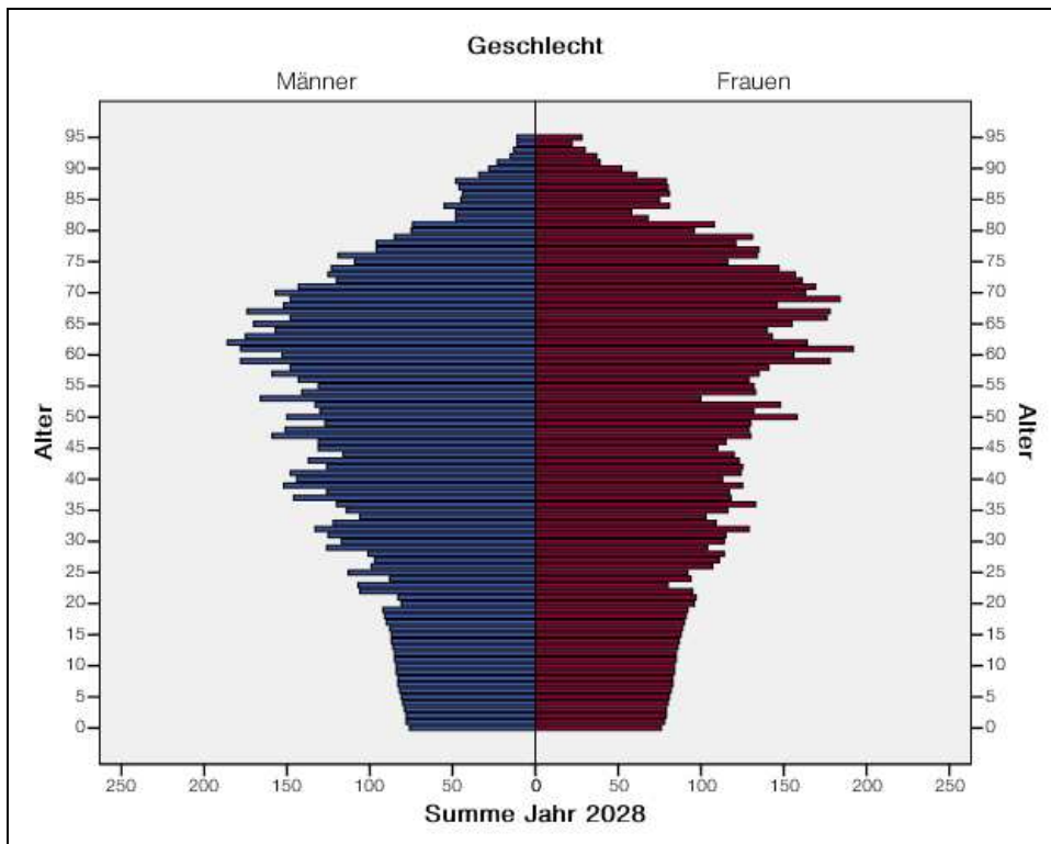
Abbildung 2: Prognose Waldkraiburg 2028
