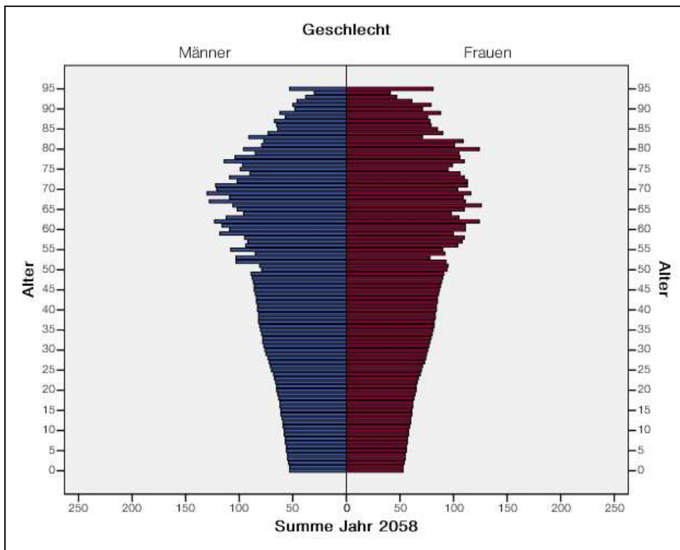
Abbildung 3: Vorausberechnung Waldkraiburg 2058
